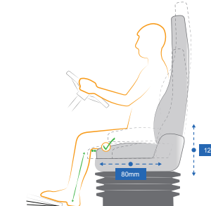
Erweiterte pneumatische Höhen- einstellung (120 mm) und Sitzkissen- tiefeinstellung (80 mm) Advanced pneu- matic height adjustment (120 mm) and seat cushion depth adjustment (80 mm)
